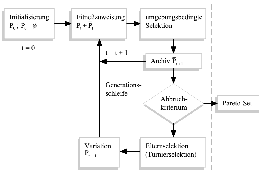
Abbildung 3: Ablaufs des evolutionären Mehrzieloptimierungsalgorithmus.
