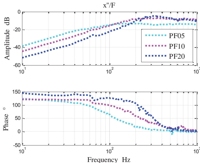
Abb. 4: Frequenzgang der im Versuch untersuchten Varianten von Strukturkoppelung durch einen Polymerpuffer. Pufferdurchmesser: PF05 – 5mm, PF10 – 10mm, PF20 – 20mm.
