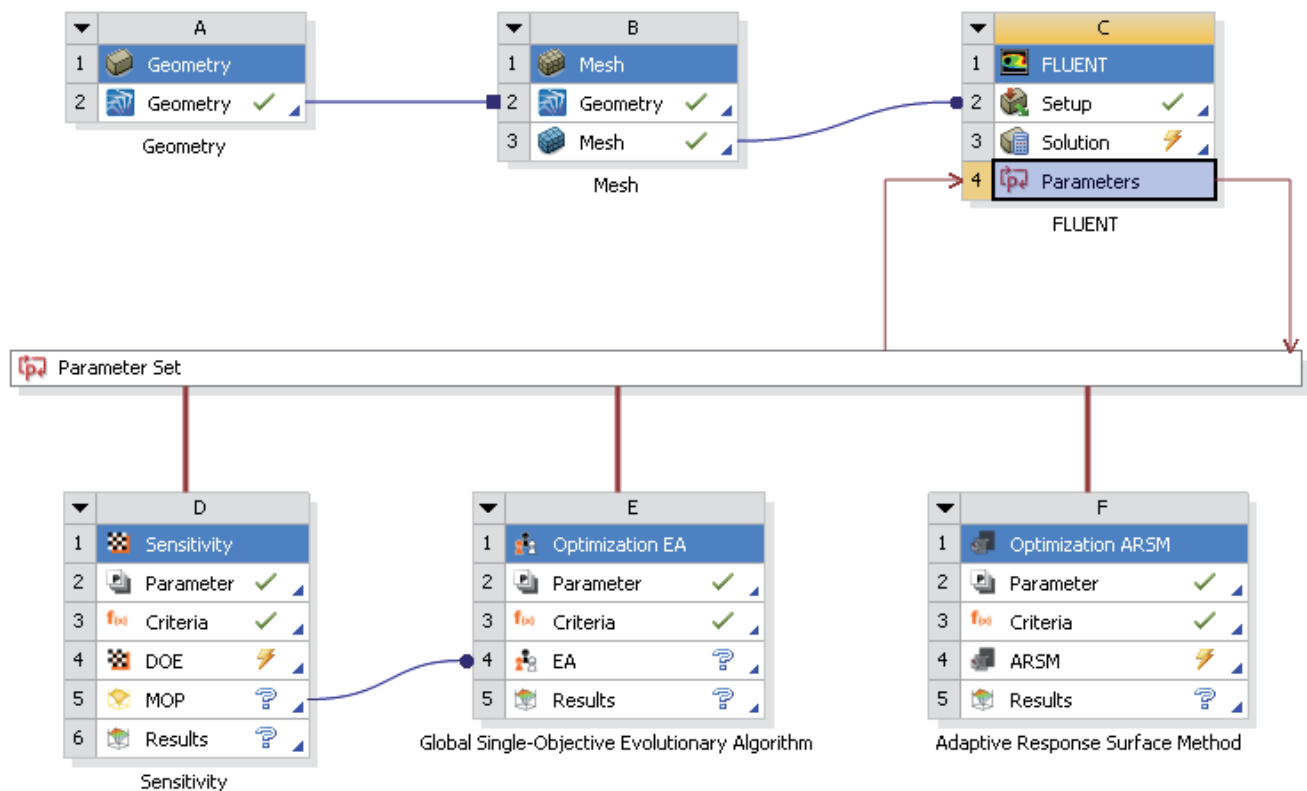
Abb. 9: Die ANSYS Workbench gekoppelt mit optiSLang inside ANSYS Workbench für das CFD-Beispiel des Raumes mit zwei Hindernissen. Anhand der Parameter aus einem CFD-Modell erfolgte nach einer Sensitivitätsanalyse eine globale Optimierung basierend auf evolutionären Algorithmen. Damit wurden einige gute Designs erzeugt, die noch nicht alle Nebenbedingungen erfüllen. Daher wurde in einem zweiten Schritt mit der Adaptiven Antwortoberflächen-Methode eine weitere, gezieltere Optimierung vorgenommen.
