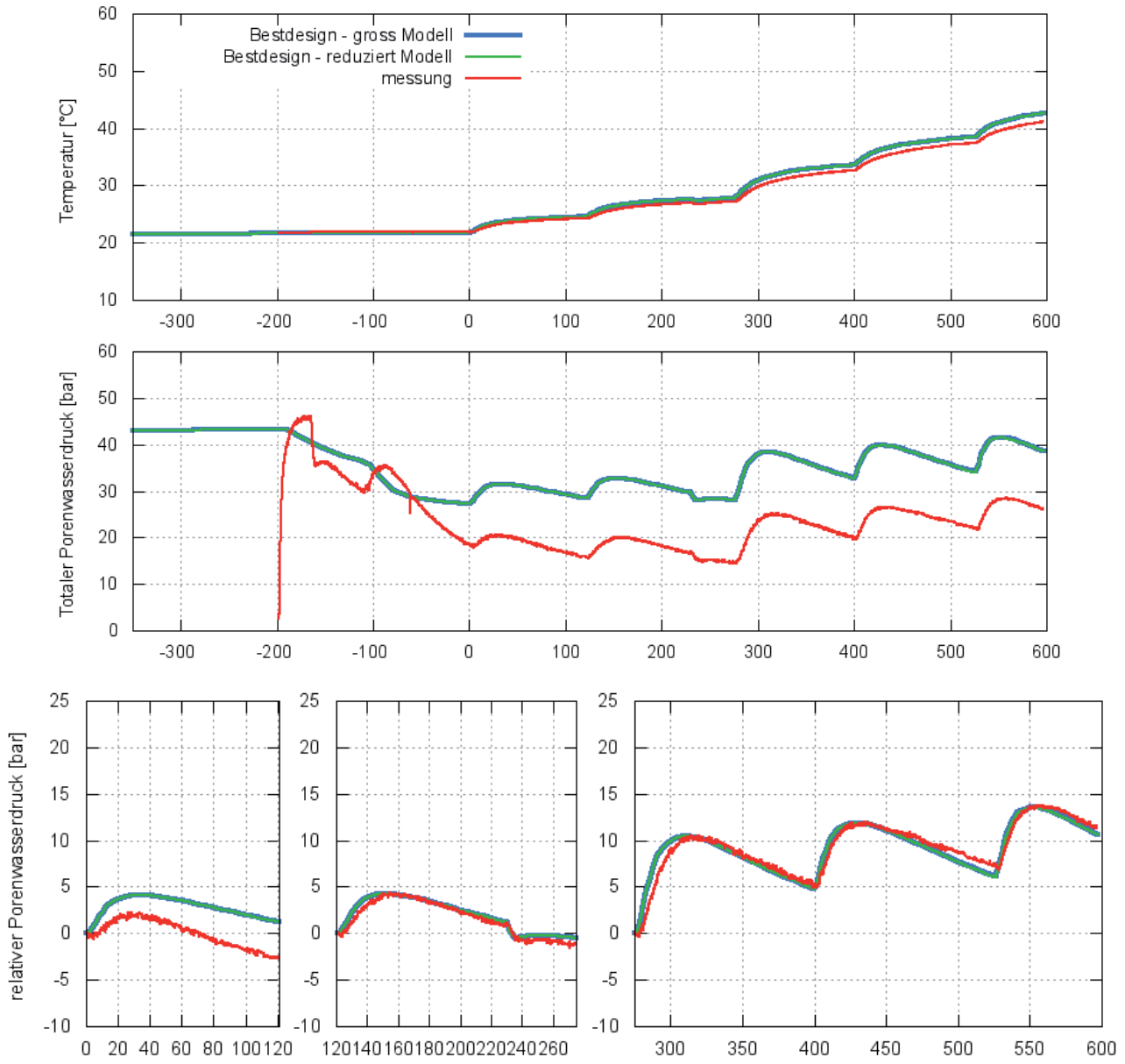
Abb. 13: Vergleich Messung vs. Simulation am Messpunkt 1252 nach der Parameteridentifikation. Oben: Temperaturverlauf, Mitte: totaler Porenwasserdruck, Unten: relativer Porenwasserdruck der drei Heizphasen.
