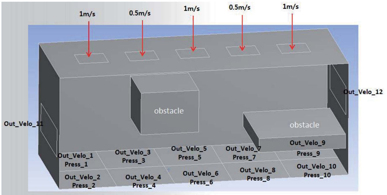
Abb. 8: Ein CFD-Beispiel eines Raumes mit zwei Hindernissen. 12 ausgangsseitige Flussgeschwindigkeiten und 10 Drücke als Eingangsparameter sind die systembeschreibenden Größen.
