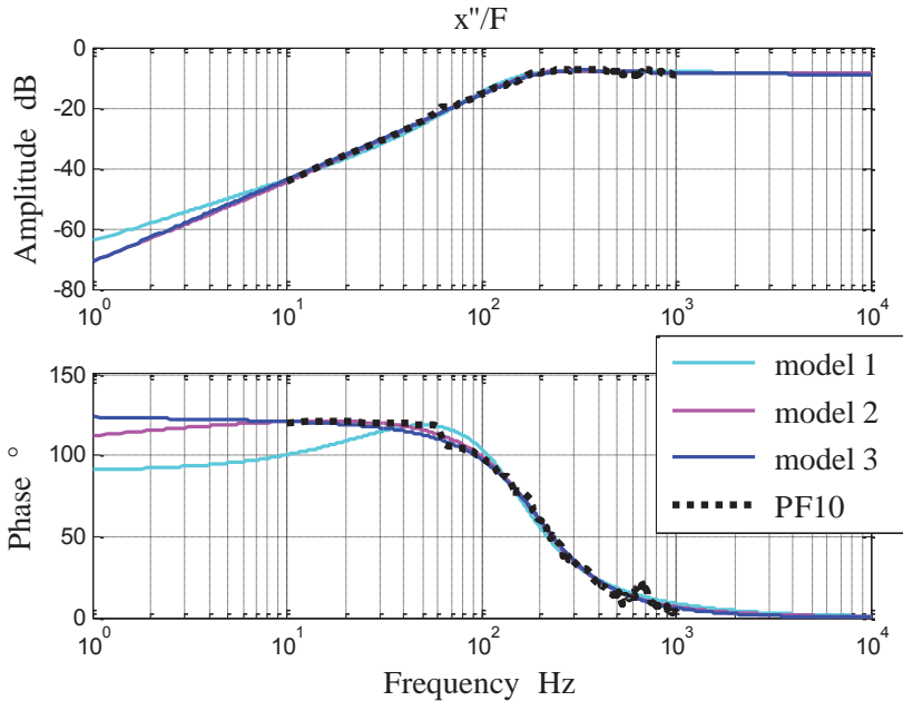
Abb. 6: Vergleich der Frequenzgänge für die Variante PF10, mit 10mm Pufferdurchmesser. model1 ist in der Formulierung mit ganzzahligen Differentialtermen gegeben durch die Gl. (4); model2 und model3 sind durch die Gl. (2) für \alpha=1/2 und für \alpha=1/3 gegeben.
