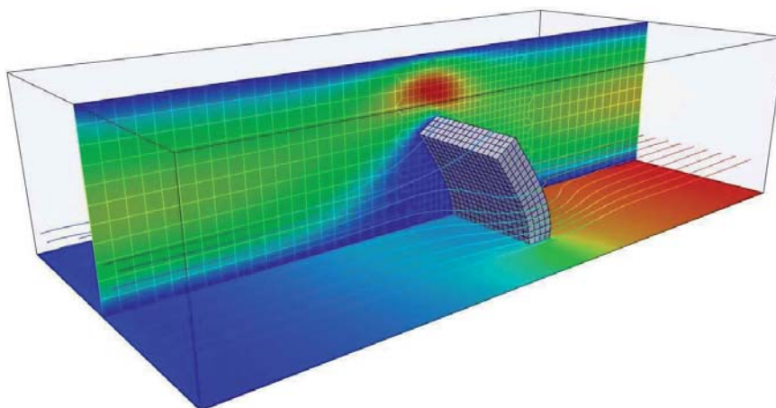
Abb. 1: Simulation einer Strömung über eine flexible wandartige Struktur [8].
