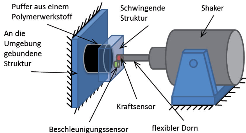
Abb. 3: Schematische Darstellung des Versuchsaufbaus.
