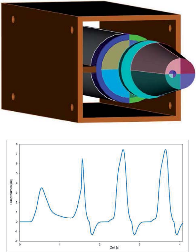
Abb. 7: Industrielles Anwendungsbeispiel Fluid-Pumpe: Geometrie in abgewandelter Form (oben) und Darstellung des simulierten Pumpvolumen für einen ausgewählten Anwendungsablauf (unten).
