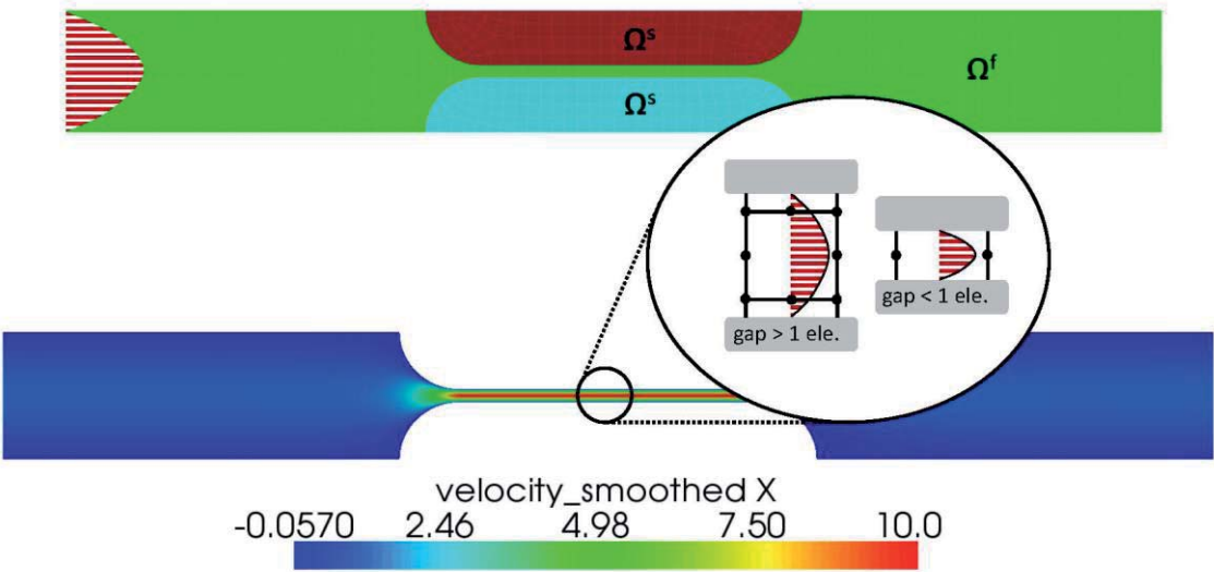
Abb. 8: Beispiel für eine Methode auf fixem Gitter zur Modellierung von Phänomenen mit einer Größenordnung kleiner als die Diskretisierungslänge (A. Popp, LNM).
